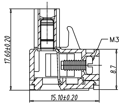
剖面图 A-A
