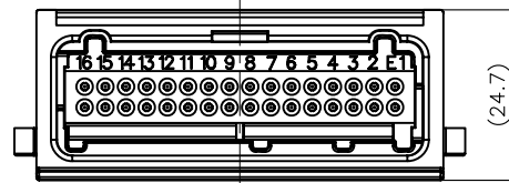
TYPE 102 CONN_ASM:12129369
