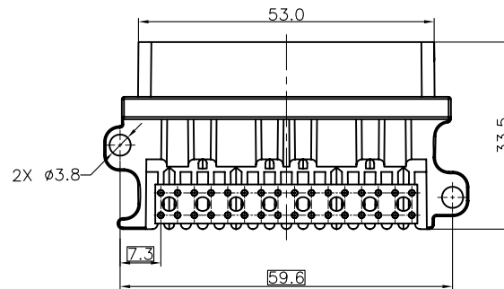
TYPE 102 CONN_ASM:12129369
