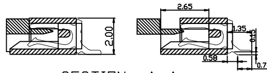
SECTION A-A
